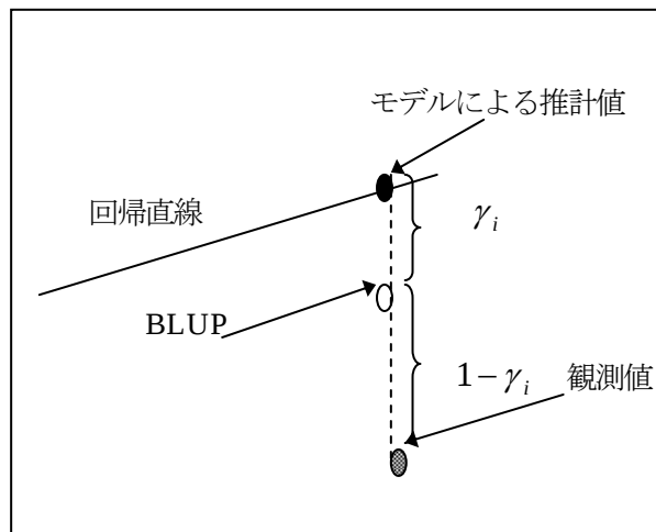
図 BLUP 推定量の意味
