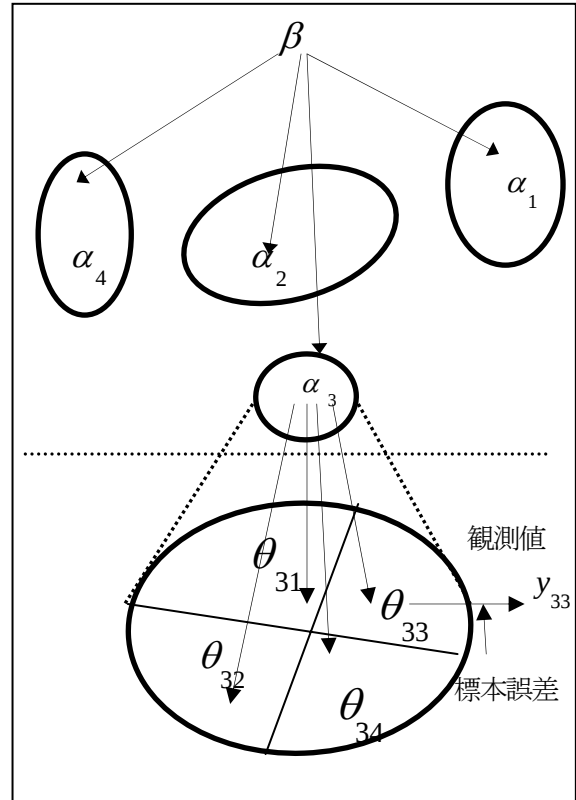
図 階層的ベイズモデルのイメージ
